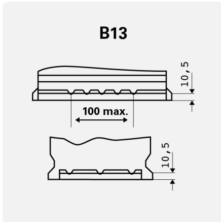
Přidrzení základny
