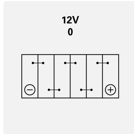
Uspořádání pólů
