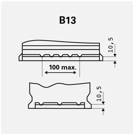
Taban tutma
